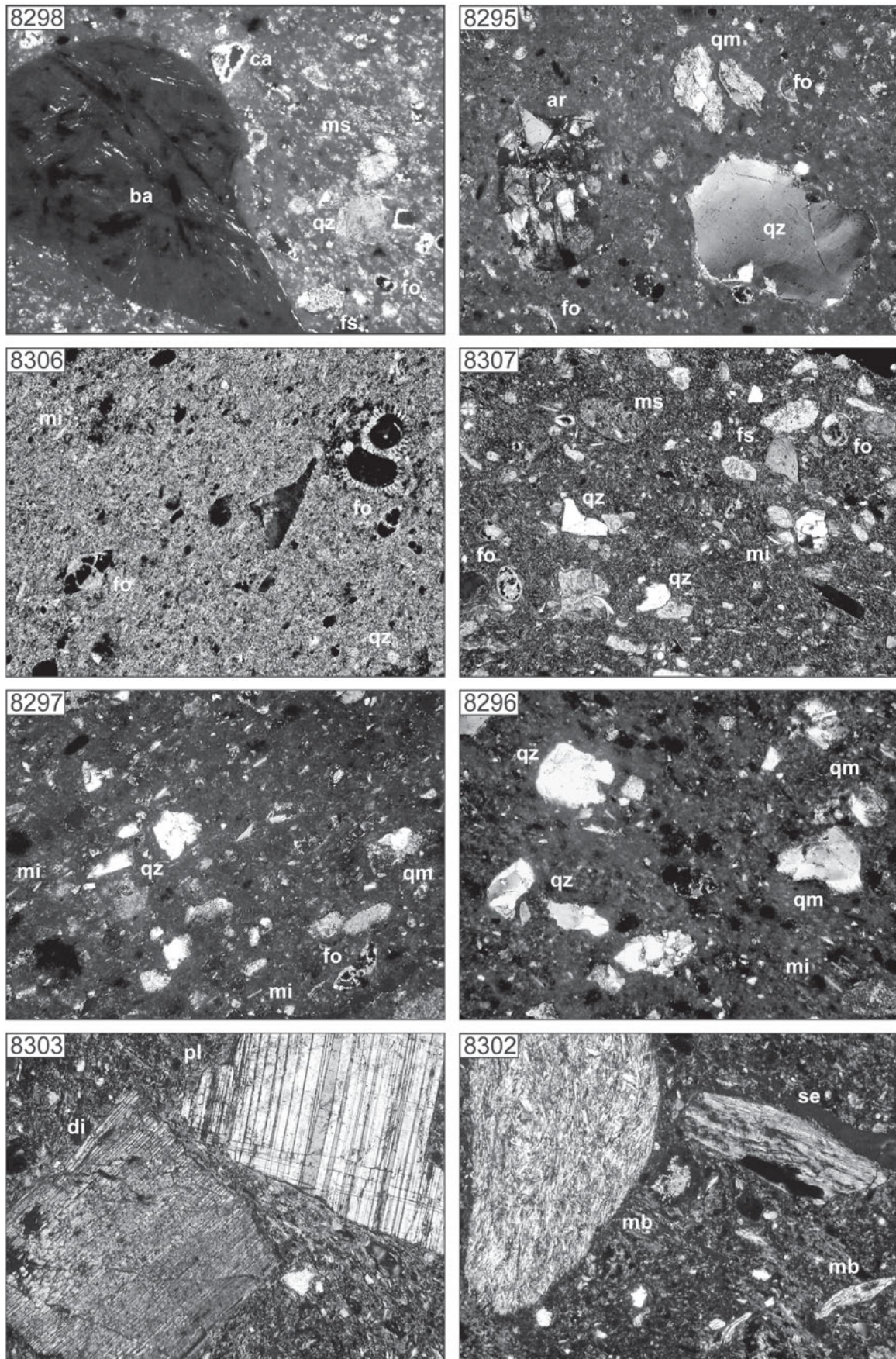
Fig. 2. Microfotografie di alcuni degli impasti analizzati (Nx, area reale: 1.3 ×1 mm); ar: arenaria, ba: basalto, ca: calcare, di: diallagio, fo: microfossile, fs: feldspato, mb: metabasite, mi: mica, ms: micascisto, pl: plagioclasio, qm: quarzomicascisto, qz: quarzo, se: serpentinoscisto.
