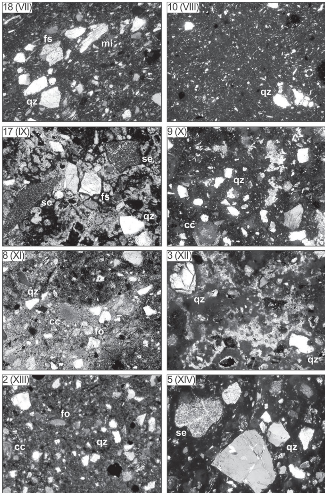
Fig. 5. Particolari in sezione sottile (Nx, area reale inquadrata: 1.3×1 mm) di alcuni dei campioni analizzati. In alto a sinistra si trovano la sigla del campione e il Gruppo petrografico di appartenenza (cf. testo); cc calcareo; fo fossile calcareo; fs feldspato; mi mica; qz quarzo; se selce.
