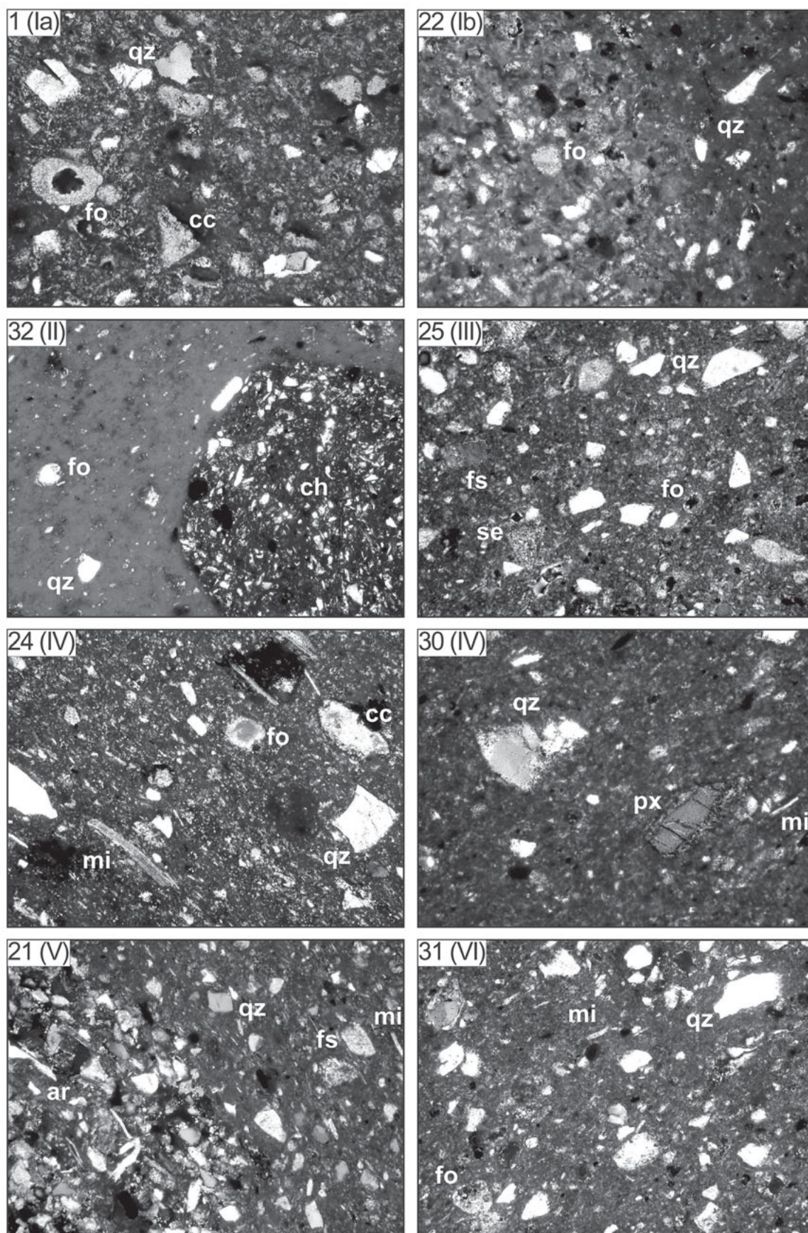
Fig. 4. Particolari in sezione sottile (Nx, area reale inquadrata: 1.3×1 mm) di alcuni dei campioni analizzati. In alto a sinistra si trovano la sigla del campione e il Gruppo petrografico di appartenenza (cf. testo); ar arenaria; cc calcare; ch chamotte; fo fossile calcareo; fs feldspato; mi mica; px clinopirosseno; qz quarzo.
